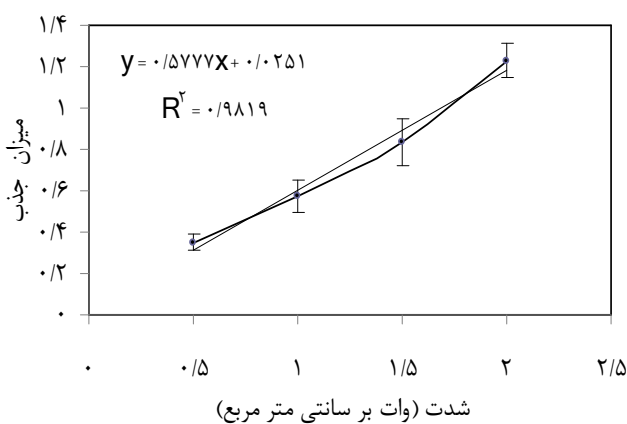
شکل ۸ نمودار تغییرات میزان جذب دزیمتر بر حسب تغییرات
