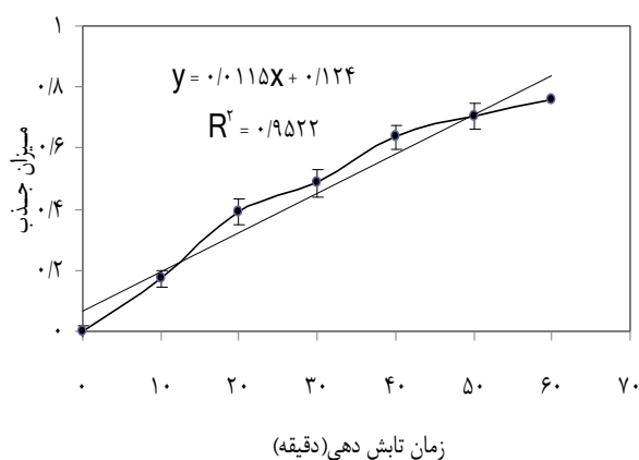
شکل ۳. منحنی شدت جذب دزیمتر در مدت زمان تابش دهی مختلف در میدان فراصوتی ۱ مگاهرتز (۲ وات بر سانتی متر مربع). تابع رگرسیون خطی و ضریب برازش در شکل ارائه شده است.
