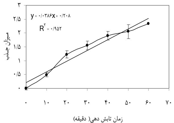
شکل ۷. منحنی تأثیر زمان تابش هم‌زمان دو میدان فراصوتی ۱
