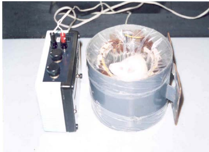
شکل ۱: نحوه پرتو دهی موش (Rat) در داخل کویل میدان مغناطیسی (شدت 2\text{ mT} با فرکانس 35\text{ Hz} ) استوانه ای به قطر و ارتفاع مؤثر به ترتیب ۹ سانتی متر و ۶ سانتی متر متشکل از چهار کلاف سولنوئید ۶۰ دوری ازسیم بیچ مسی به قطر 0.55 میلی متر.
