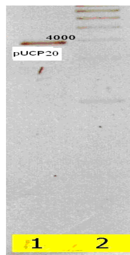
شکل ۴: الف: باندهای حاصل پس از اولتراکلین باندهای مربوط به پلاسمید پس از استخراج با روش لیز قلیایی pUCP20 (چاهک شماره ۱)، مارکر (چاهک شماره ۲).
